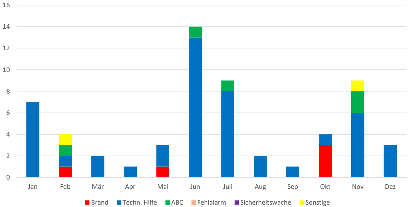
Monatliche Einsatzverteilung 2021
